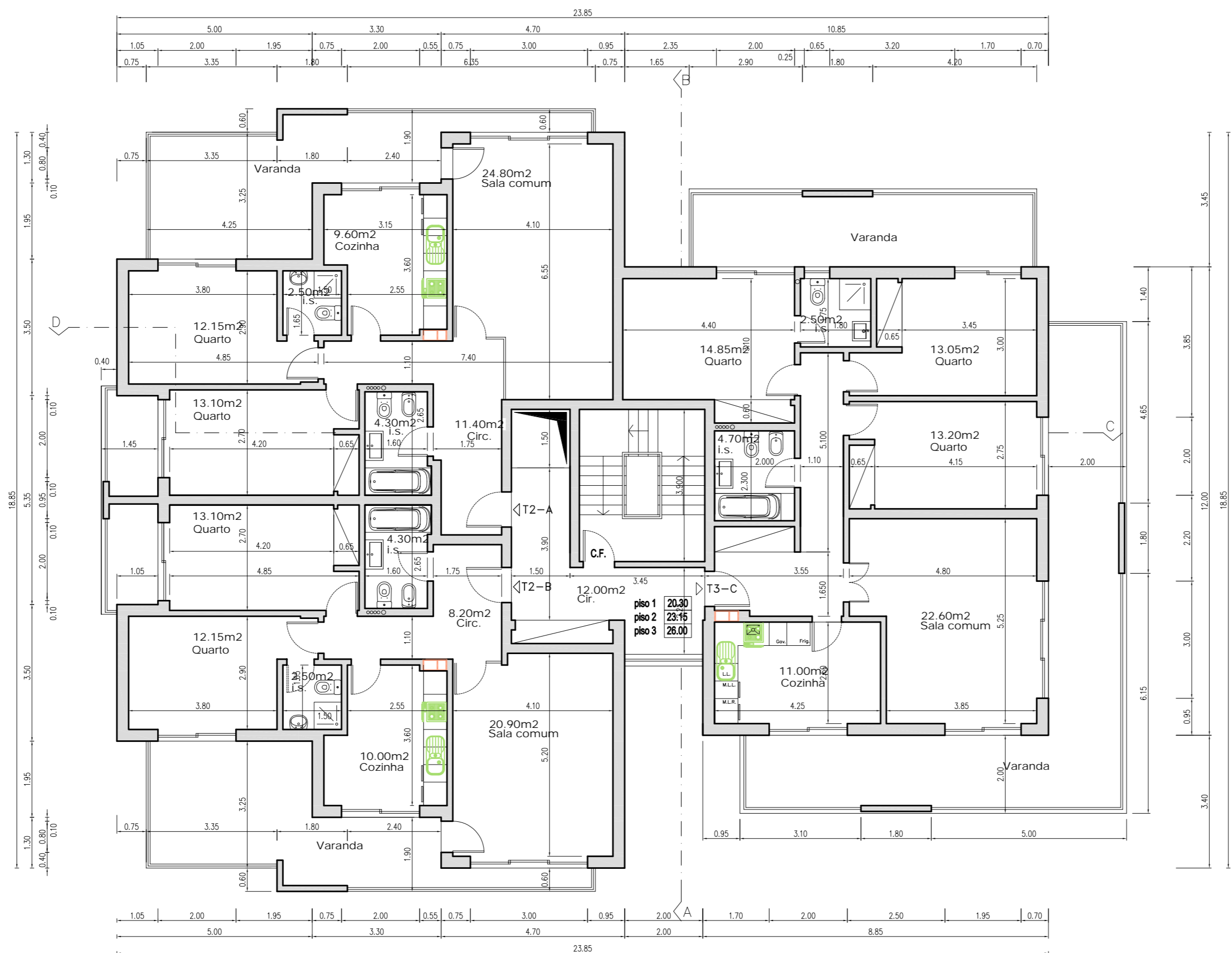
PLANTA DOS PISOS 1, 2 e 3
